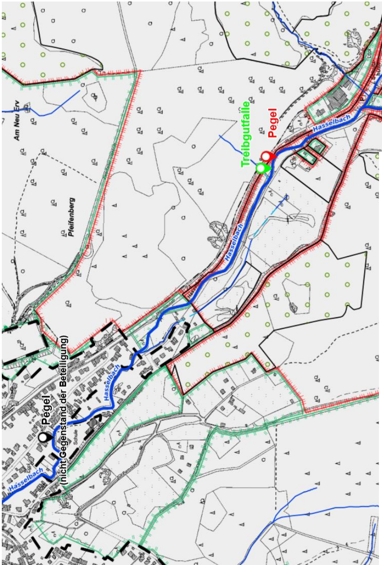
Abb. 1: Übersicht über die Lage der geplanten Pegel und Treibgutfaule.
